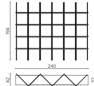
ET 2400 bookshelf 240cm libreria 240cm étagère 240cm
