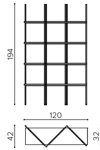
ET 1200 bookshelf 120cm libreria 120cm étagère 120cm
