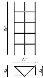
ET 0800 bookshelf 80cm libreria 80cm étagère 80cm
