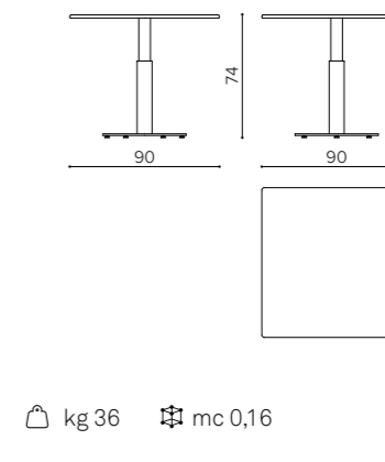
IS 9090 Table 90x90x74 cm Tavolo 90x90x74 cm Table 90x90x74 cm
