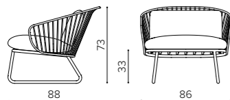
NT 1000 OUT outdoor armchair with cushions poltrona da esterni con cuscini fauteuil d'extérieur avec coussins
