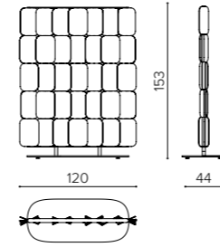
PA 1215 acoustic panel pannello acustico séparateur acoustique
