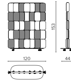
PA 1215R MIX acoustic panel with castors pannello acustico con ruote séparateur acoustique avec roues
