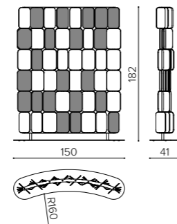
PA 1518C MIX curved acoustic panel pannello acustico curvo séparateur acoustique courbé
