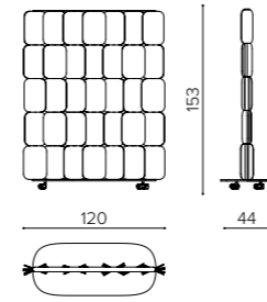
PA 1215R acoustic panel with castors pannello acustico con ruote séparateur acoustique avec roues
