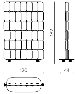
PA 1218R acoustic panel with castors pannello acustico con ruote séparateur acoustique avec roues
