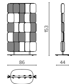
PA 0815 MIX acoustic panel pannello acustico séparateur acoustique
