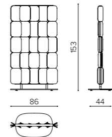
PA 0815 acoustic panel pannello acustico séparateur acoustique
