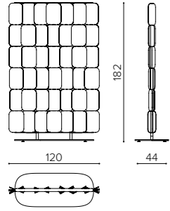
PA 1218 acoustic panel pannello acustico séparateur acoustique
