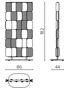
PA 0818 MIX acoustic panel pannello acustico séparateur acoustique
