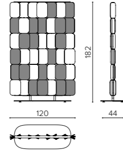
PA 1218 MIX acoustic panel pannello acustico séparateur acoustique
