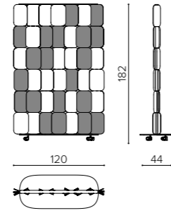
PA 1218R MIX acoustic panel with castors pannello acustico con ruote séparateur acoustique avec roues
