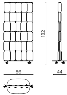
PA 0818R acoustic panel with castors pannello acustico con ruote séparateur acoustique avec roues
