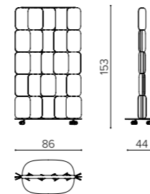
PA 0815R acoustic panel with castors pannello acustico con ruote séparateur acoustique avec roues
