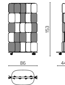
PA 0815R MIX acoustic panel with castors pannello acustico con ruote séparateur acoustique avec roues
