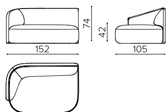
SY 150L/R right 2-seater module modulo a 2 posti destro module 2 places droit
