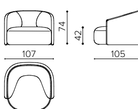
SY 1000 armchair poltrona fauteuil
