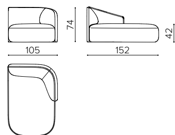
SY 1P00L/L left peninsula module modulo penisola sinistro module péninsule gauche
