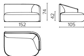
SY 150L/L left 2-seater module modulo a 2 posti sinistro module 2 places gauche
